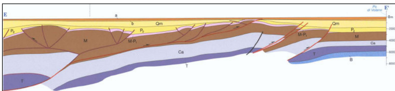
Figura 6 – Carta Sismotettonica dell'Emilia Romagna (RER – CNR, 2004)
